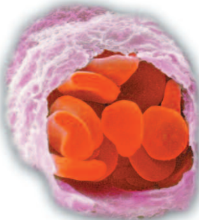
Krvne ćelije
