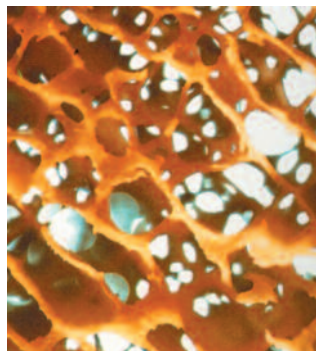
Koštana srž
